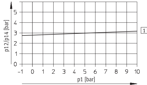
MVH-5/3...-1/4-S-B
