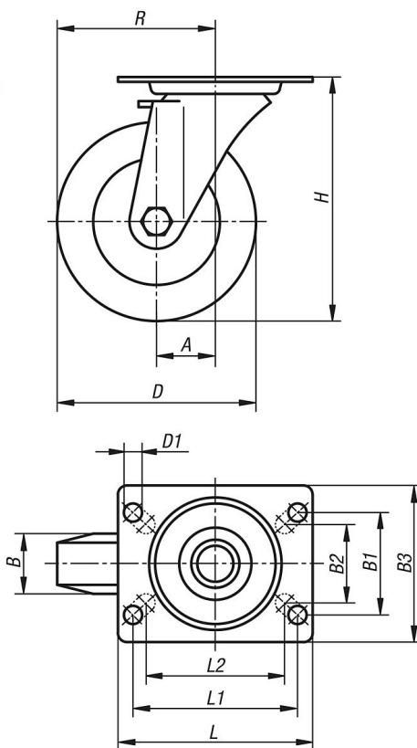
Lenkrolle
